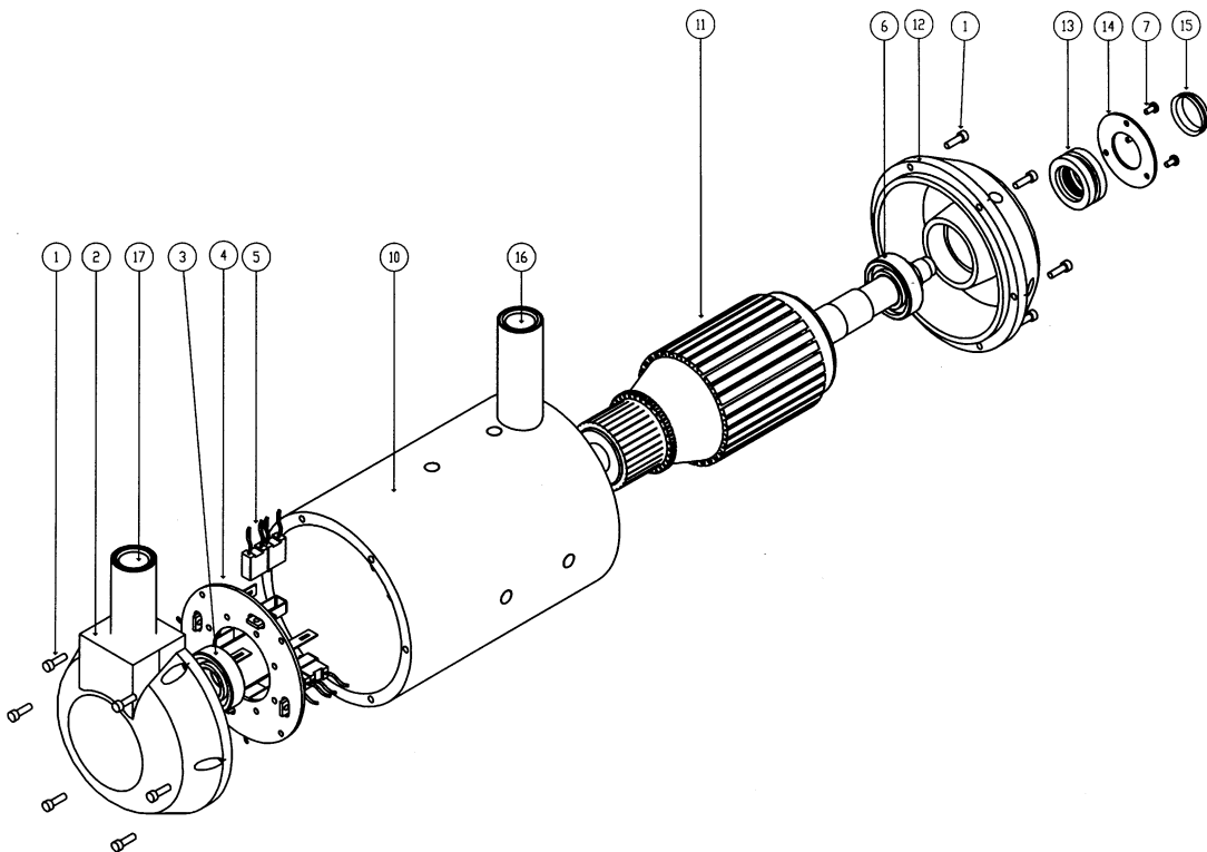
Tekening 8.2 CP90
