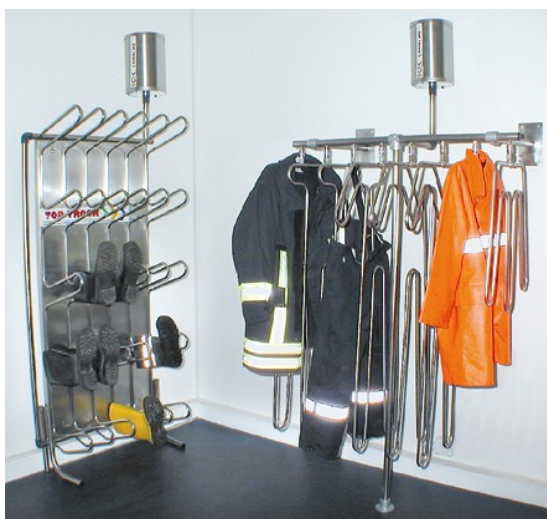
Système de séchage, montage mural ou sur pieds
